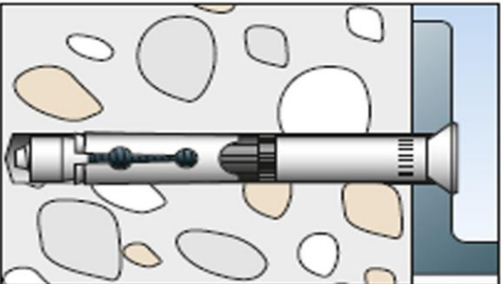
3. Insert anchor bolt.
