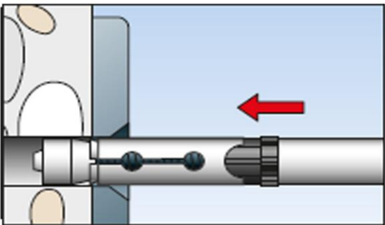
3. Insert anchor bolt.
