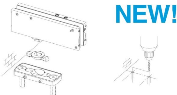
fissaggio nuova piastra - new plate fixing
